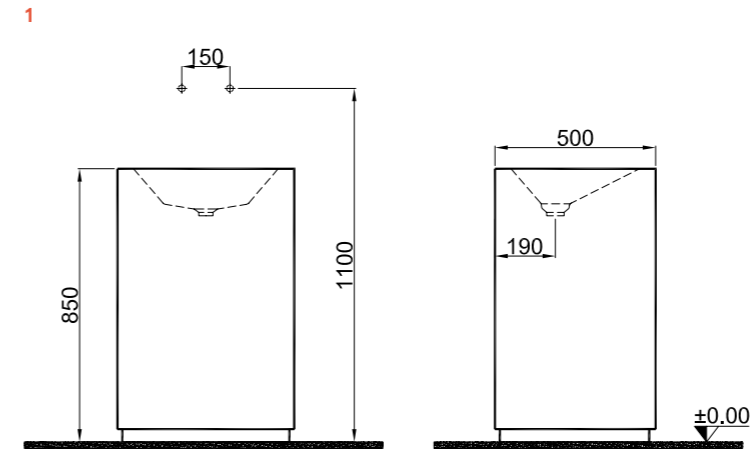
K-3 Standalone Ön ve Yan Görünüş / K-3 Standalone Front and Side View
